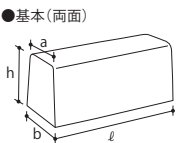
両面歩車道タイプ寸法 (洗い出し/擬石仕上げ)
