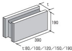
■オール充填用 (横筋)
