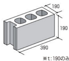
■コーナー用 (C種)
